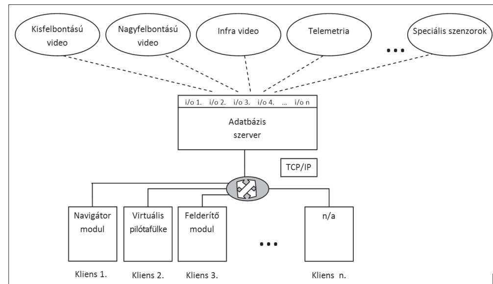
5. ábra. Az AirGuardian földi szoftverrendszerének logikai vázlata
